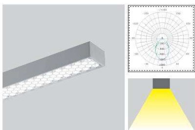
SJ-中间背盒吊装 SJ-Suspended
