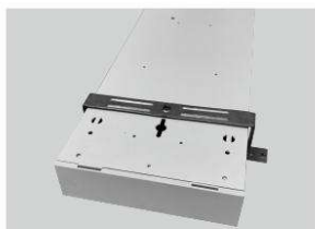
R-无边嵌装配置
